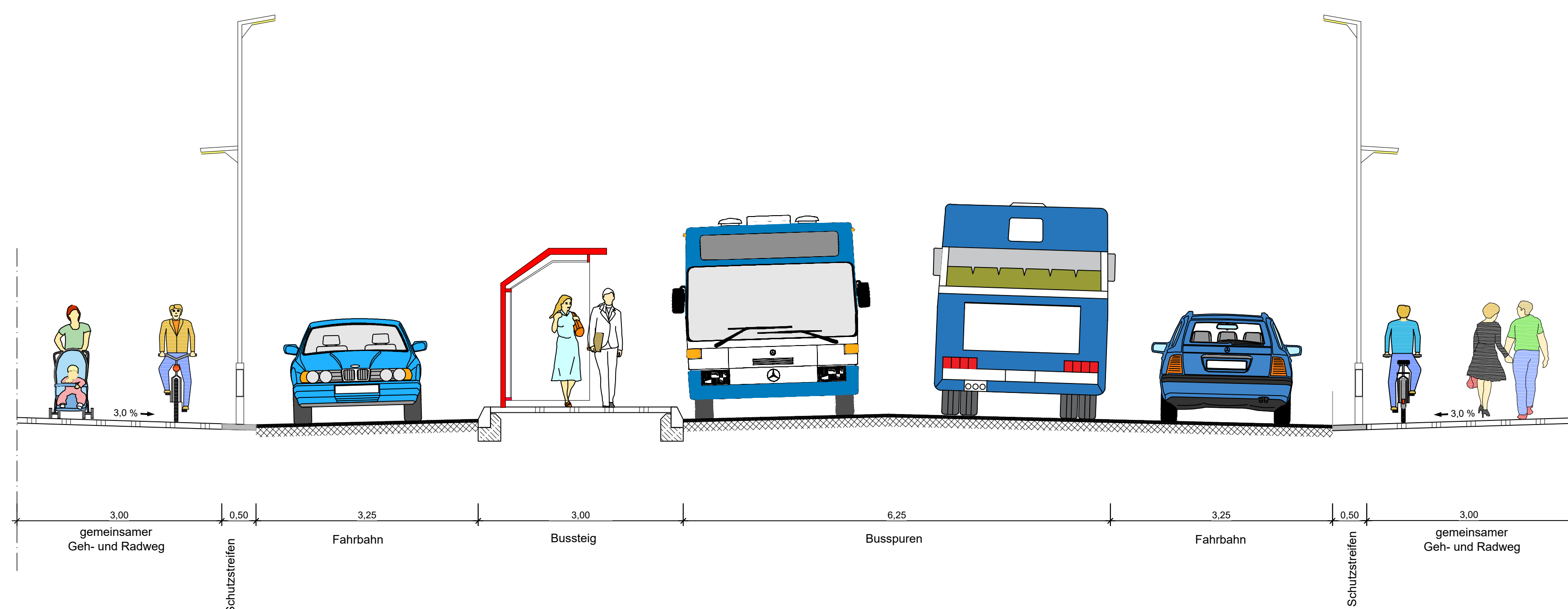
Querschnitt A - A
